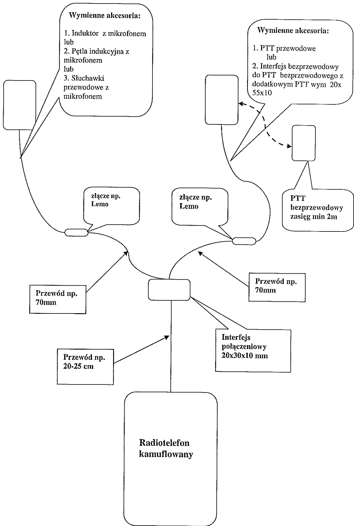
Schemat połączeń akcesoriów kamuflowanych.
