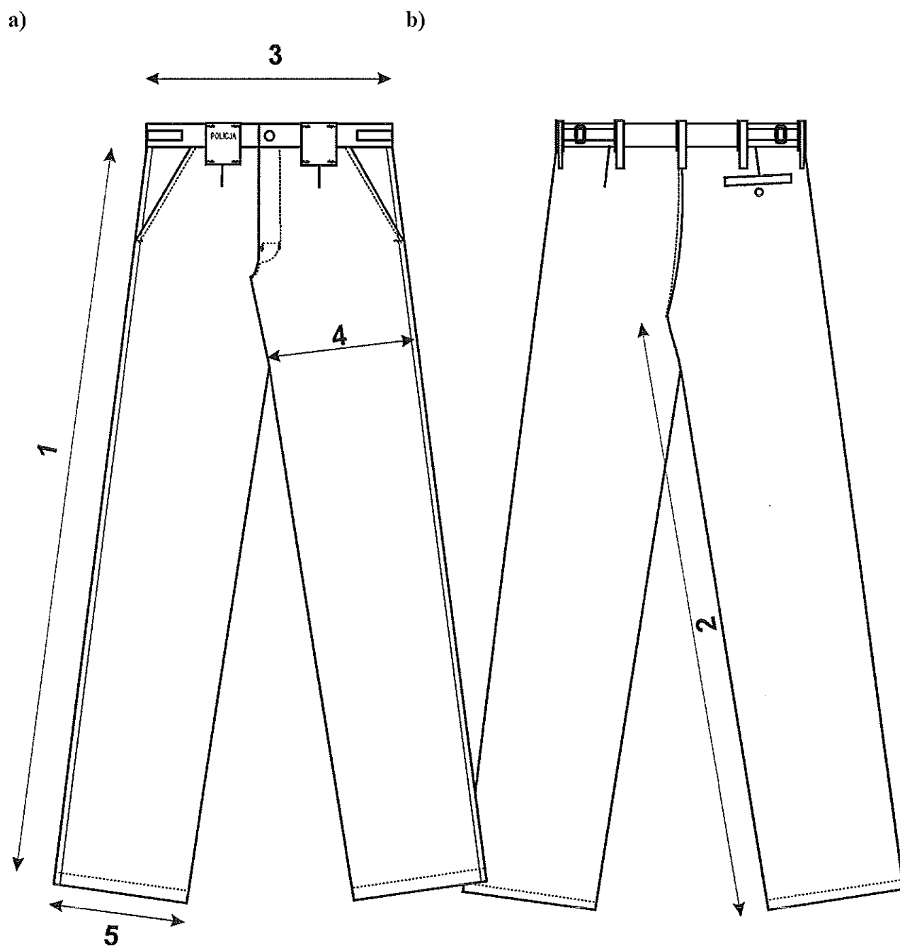
Rys. 3. Rysunek spodni służbowych letnich do półbutów: a) przód, b) tył.
