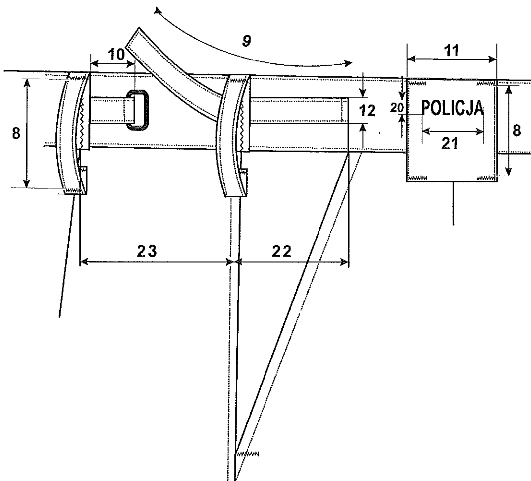
Rys. 5. Rysunek spodni służbowych letnich do półbutów – pasek.
