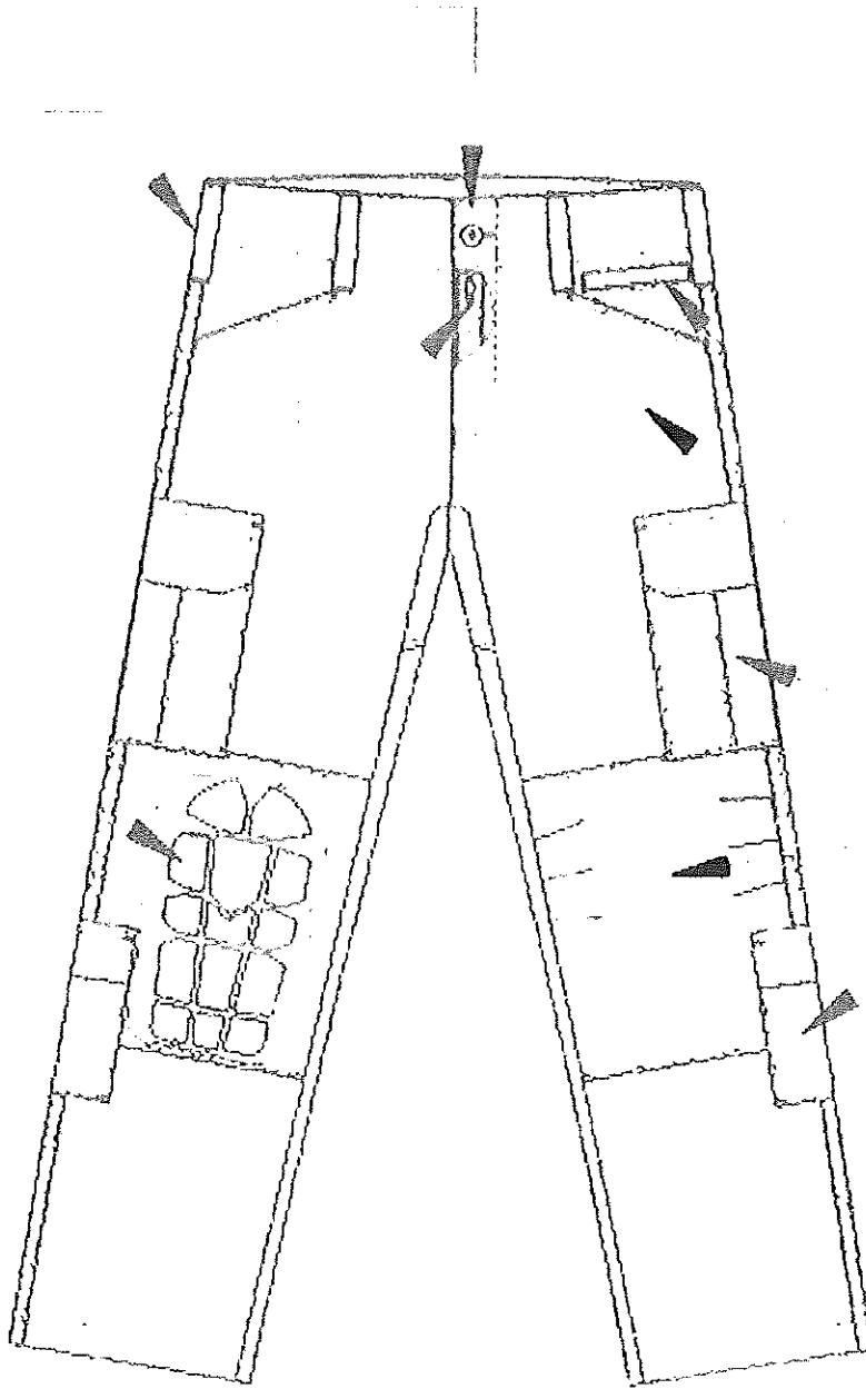
Rys. 4. Spodnie munduru letniego – elementy składowe – widok z przodu.
