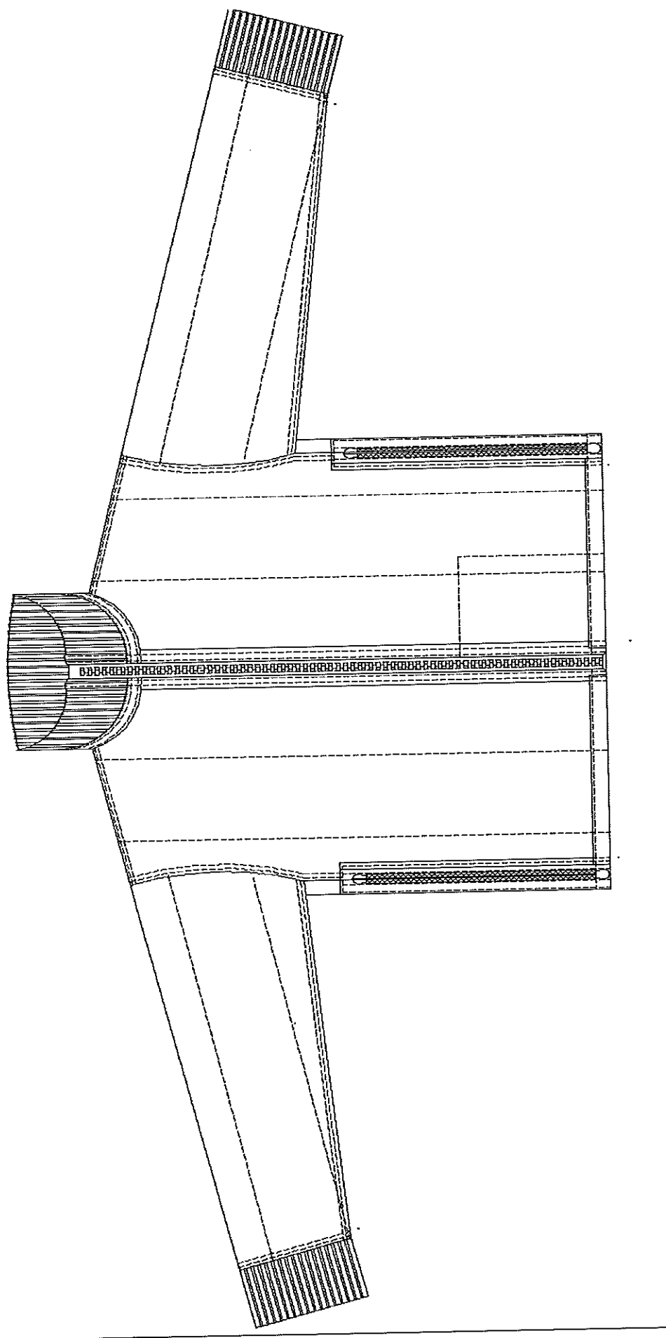
Rys. 9. Podpinka ocieplająca przód – spód
