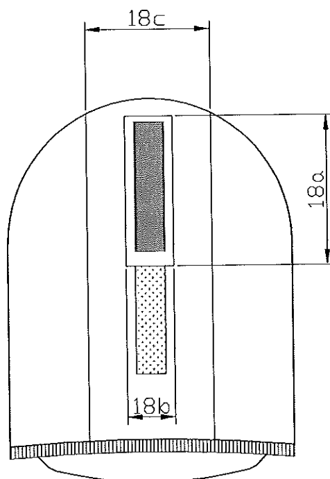
Rys. 16. Kurtka służbowa zimowa – kaptur tył – wierzeh
