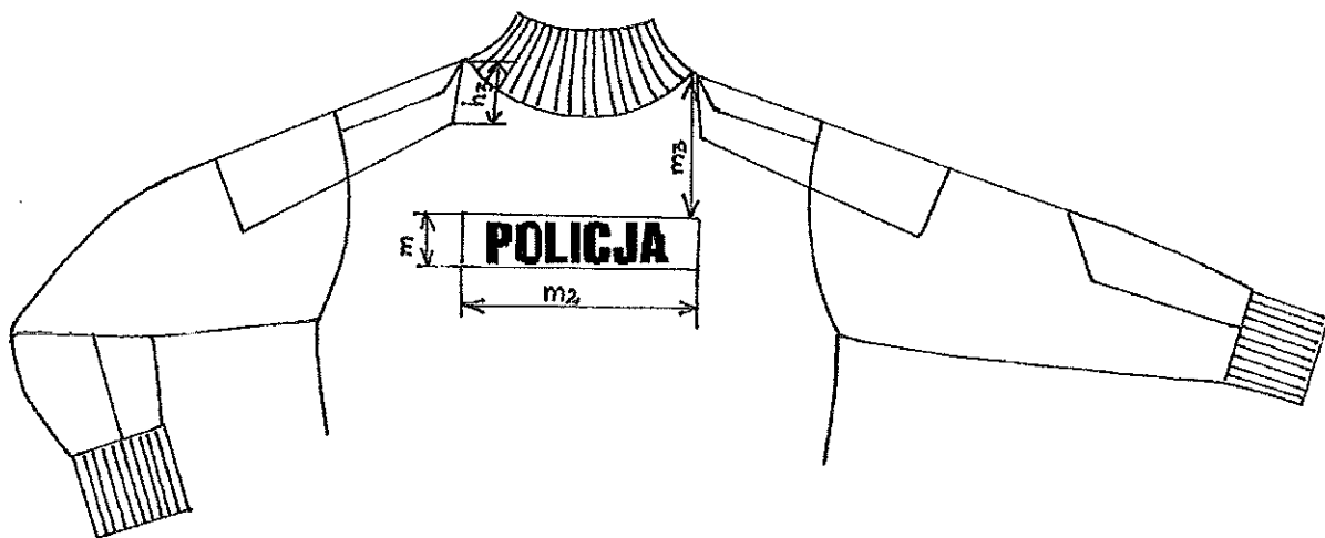
Rys. 3. Sweter służbowy – przód i tył. Wymiarowanie
