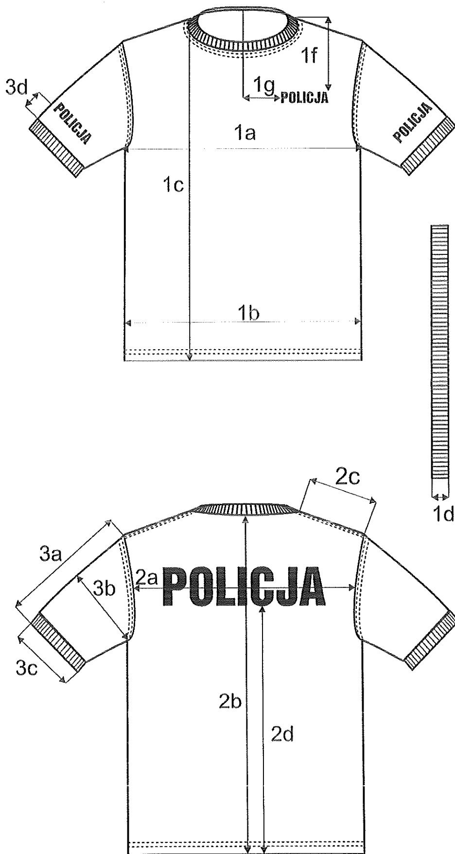
Rys. 2. Koszulka z krótkim rękawem T-shirt. Wymiarowanie.
