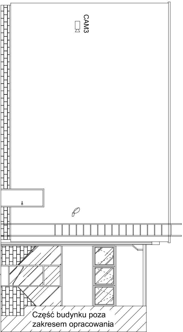
Elewacja C
