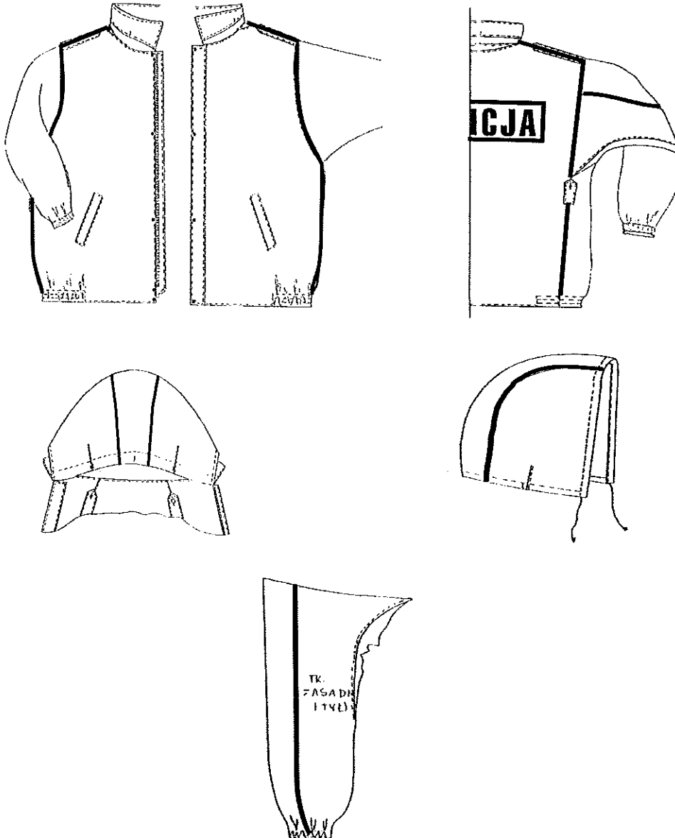
Rys. 19. Kurtka – miejsca klejenia
